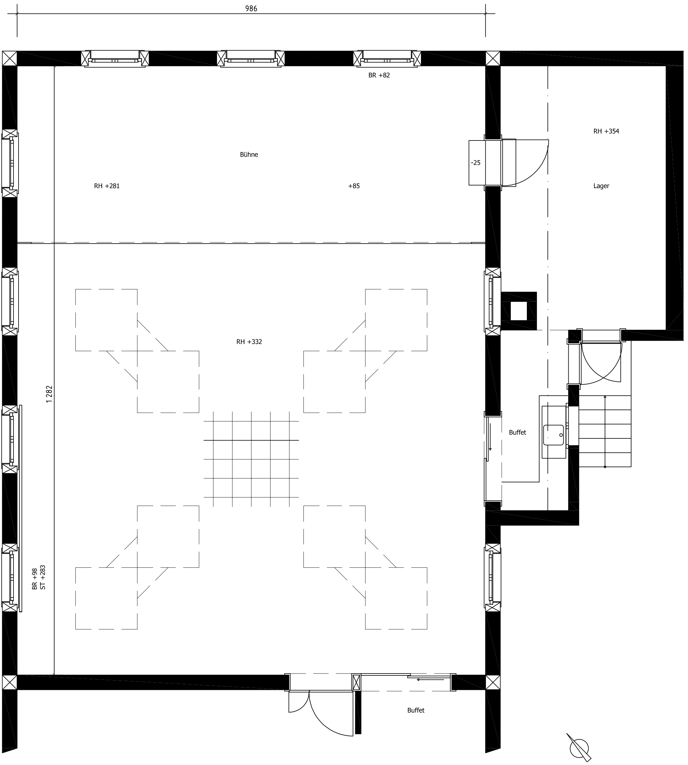
Restaurant Bahnhof, Bigenthal Grundriss Eventsaal mit Bühne Masstab 1:50, T. Oberli, März 2015
